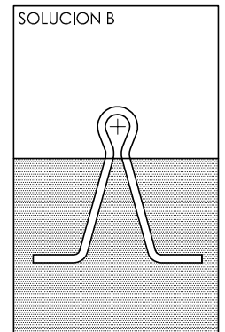
DETALLE: GUIA INFERIOR (2 modelos: A o B)
